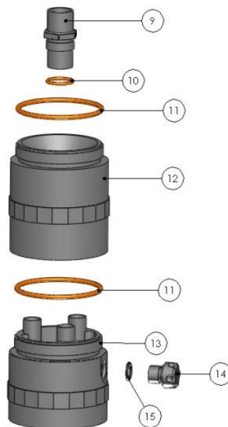
PM 10 Impactor Assembly PN 520-000
